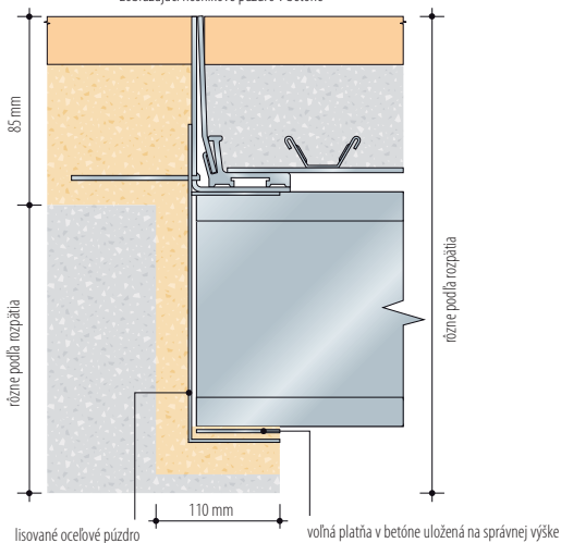
Sekcia AA
