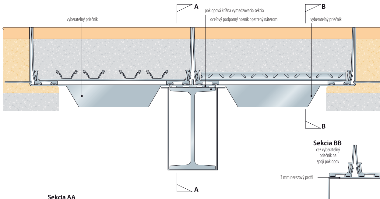
Sekcia AA
